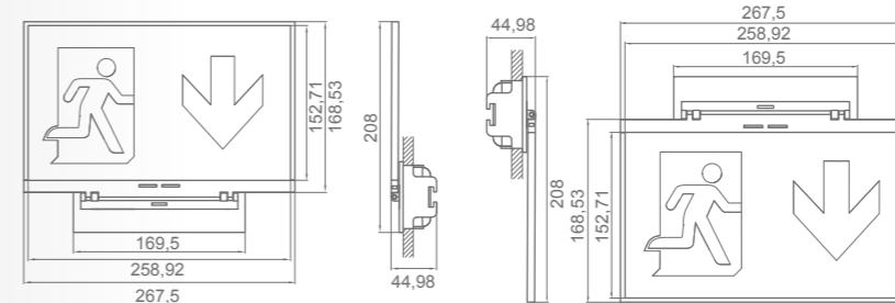
Empotrada pared
