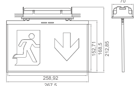
Empotrada techo
