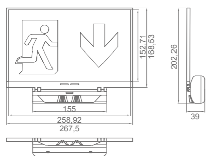
Superficie pared
