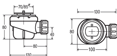
MACALPINE 70. 0,5L/S
