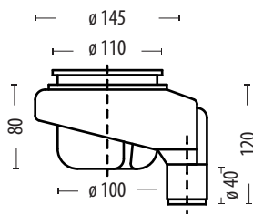
VIEGA 80 VERTICAL. 0,64L/S
