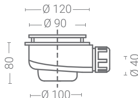
GEBERIT 80. 0,5L/S
