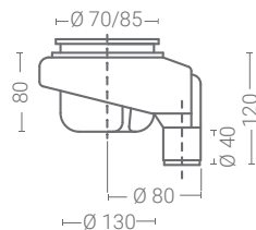
MACALPINE 50. 0,5L/S
