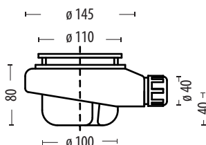
GEBERIT 80. 0,5L/S
