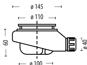
VIEGA 60 HORIZONTAL. 0,55L/S
