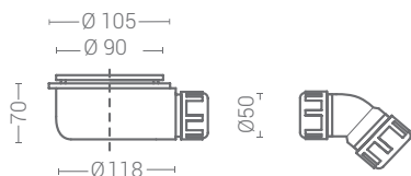
MACALPINE 70. 0,5L/S
