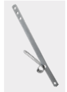
Palanca PA 30 Ref. 0154007030 Granel 25 uds/caja PVP: 0,85 € Longitud: 300 mm
