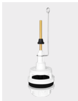
DESCARGADOR DC 261 Ref. 0156004810 Packaging Bolsa 25 uds/caja PVP: 3,05 € Ø 5 mm + Longitud: 165 mm (Latón) Base: PS/SBR (Plástico)
