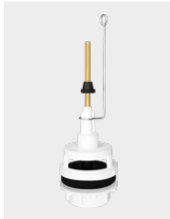
DESCARGADOR DC 71 Ref. 0156002210 Packaging Bolsa 25 uds/caja PVP: 3,30 € Ø 7 mm + Longitud: 165 mm (Latón) Base: PS/SBR (Plástico)
