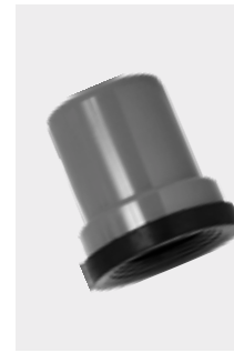
Manguito M 11 Ref. 0138043020 Granel 36 uds/caja PVP: 4,50 € Recto Ø 110 mm
