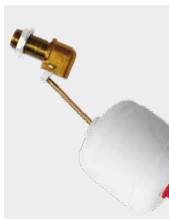
GCB 1 Ref. 0151650630 Packaging Bolsa 25 uds/caja PVP: 5,50 € Grifo lateral (Latón) + Tuerca + Boya Ø 3/8" Latón + Longitud: 30 mm
