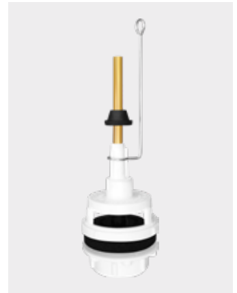
DESCARGADOR DC 251 Ref. 0156003510 Packaging Bolsa 25 uds/caja PVP: 4,45 € Ø 12 mm + Longitud: 175 mm (Latón) Base: PS/SBR (Plástico)
