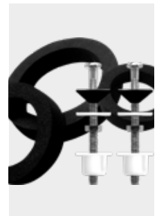
Kit Juntas KJT 1 Ref. 0138576010 Packaging Bolsa 10 uds/caja PVP: 3,20 € Ø 111 / 82 / 56 mm x 15 Espesor
