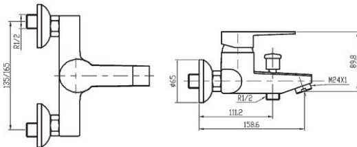
Mezclador exterior con inversor baño-ducha. Exterior mixer tap with bath-shower selector. Mitigeur bain douche avec inverseur.
