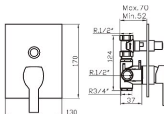
Monomando baño-ducha empotrado. Concealed bath-shower. Mitigeur bain-douche à encastrer.
