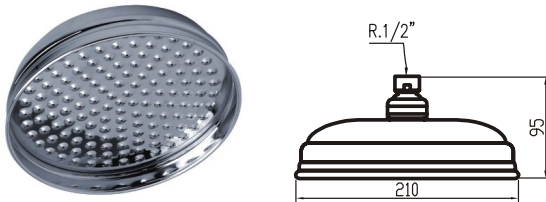
Rociador TERRA. Shower sprayer TERRA. Asperseur TERRA.
