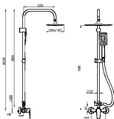
Mezclador exterior para ducha, con barra vista fija. Shower mixer, with fixed view bar. Mitigeur de douche d'extérieur, avec barre de vision fixe.
