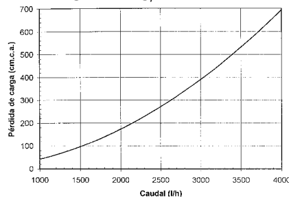
VÁLVULA DE 3/4"
